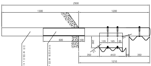
가드레일 설치도
