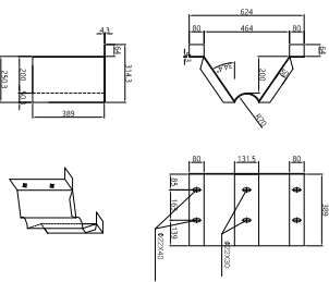
블럭아웃 상세도
