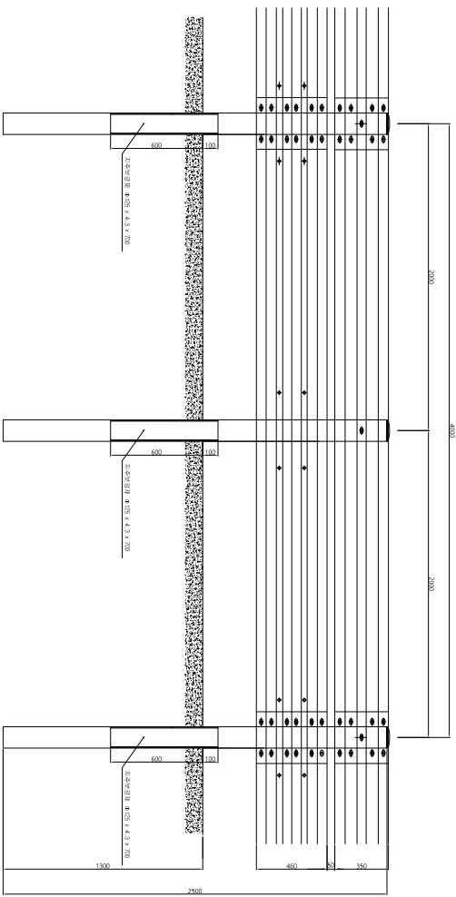
가드레일 설치도
