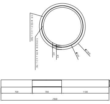
지주 상세도
