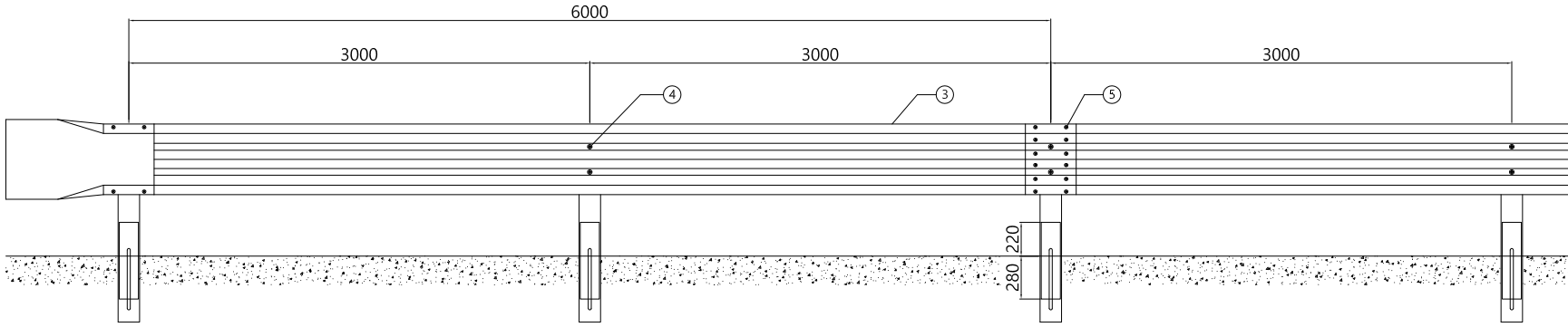
⊕ 레일
