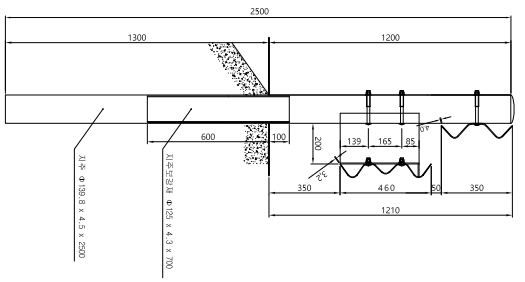
가드레일 설치도
