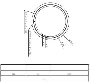
지주 상세도
