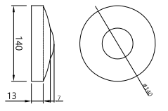
지주 덮개 상세도
