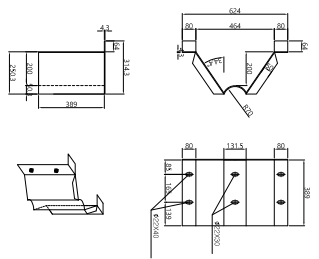
블럭아웃 상세도
