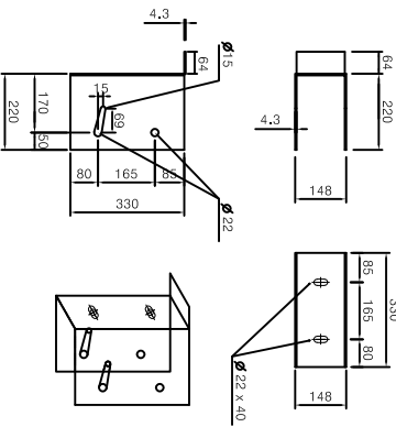
블럭아웃상세도
