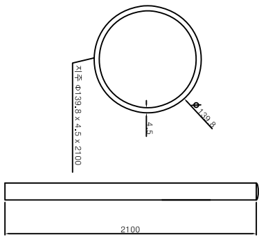
지주 상세도
