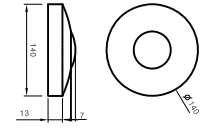
지주 덮개 상세도
