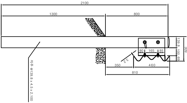
레일고정 B/N
